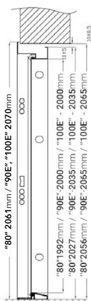
POZIOM 0 POSADZKA
